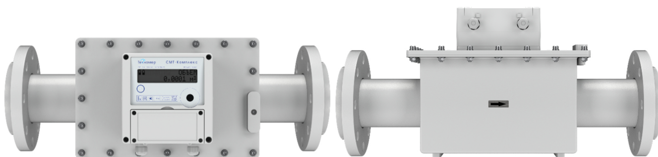
Рисунок 23 – Общий вид счетчиков газа микротермальных СМТ-Комплекс-G40-2, СМТ-Комплекс-G65, СМТ-Комплекс-G100
