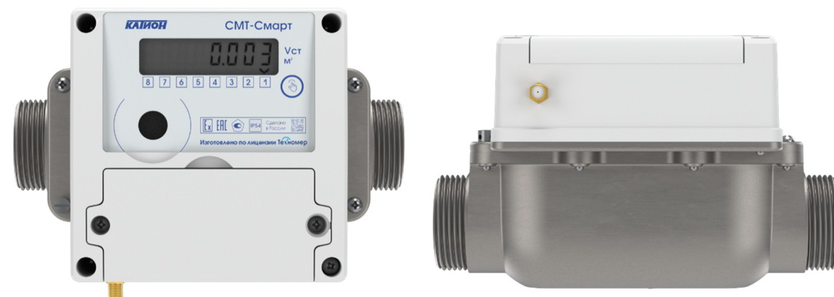
Рисунок 12 – Общий вид счетчиков газа микротермальных CMT-Смарт G4-B, CMT-Смарт G6-B изготовленных ООО «ПО «КАТИОН»
