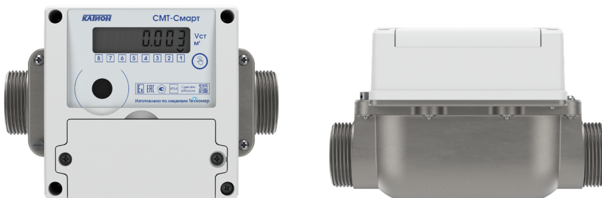
Рисунок 10 – Общий вид счетчиков газа микротермальных CMT-Смарт G4, CMT-Смарт G6 изготовленных ООО «ПО «КАТИОН»
