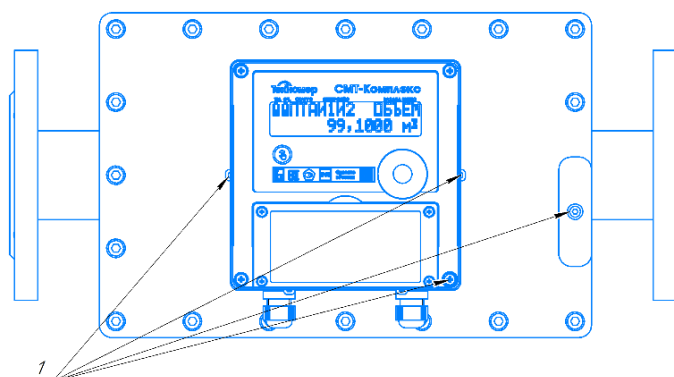
Исполнение СМТ-Комплекс типоразмеров G40, G40-2, G65, G100
