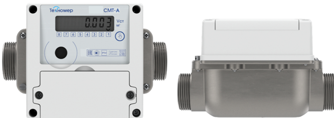
Рисунок 1 – Общий вид счетчиков газа микротермальных CMT-A G4, CMT-A G6 изготовленных ООО «Техномер»
