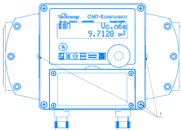
Исполнение СМТ-Комплекс, СМТ-Комплекс-К, СМТ-Комплекс-ДКЗ типоразмеров G4 – G25
