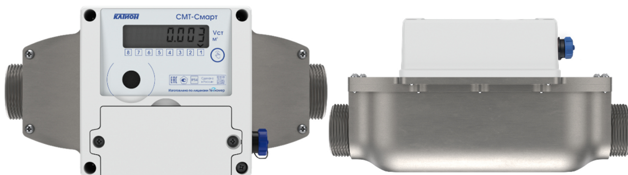
Рисунок 18 – Общий вид счетчиков газа микротермальных СМТ-Смарт-ДКЗ-G4, СМТ-Смарт-ДКЗ-G6, СМТ-Смарт-ДКЗ-G10 изготовленных ООО «ПО «КАТИОН»
