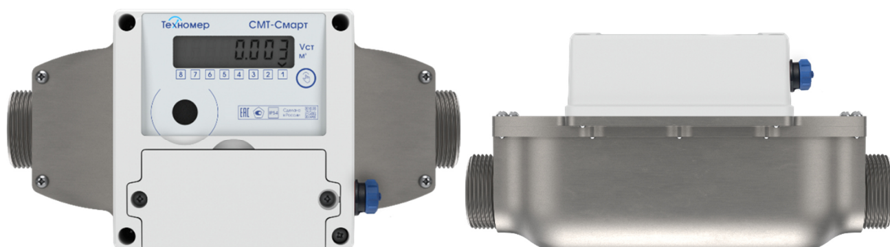
Рисунок 17 – Общий вид счетчиков газа микротермальных СМТ-Смарт-ДКЗ-G4, СМТ-Смарт-ДКЗ-G6, СМТ-Смарт-ДКЗ-G10 изготовленных ООО «Техномер»
