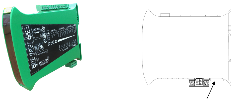
Разрушаемая наклейка, закрывающая доступ к разъемам сигнальных кабелей (кабелей питания) и предотвращающая несанкционированный доступ для замены УОАД
