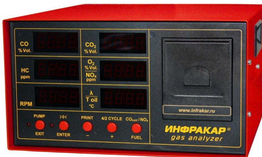
Рисунок 4 – Общий вид газоанализаторов ИНФРАКАР в экспортном исполнении (вид спереди)
