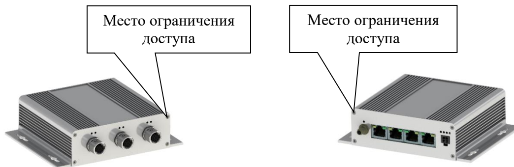
д) выносной электронный блок DMU/AMU/блок согласования нагрузки PSBU
