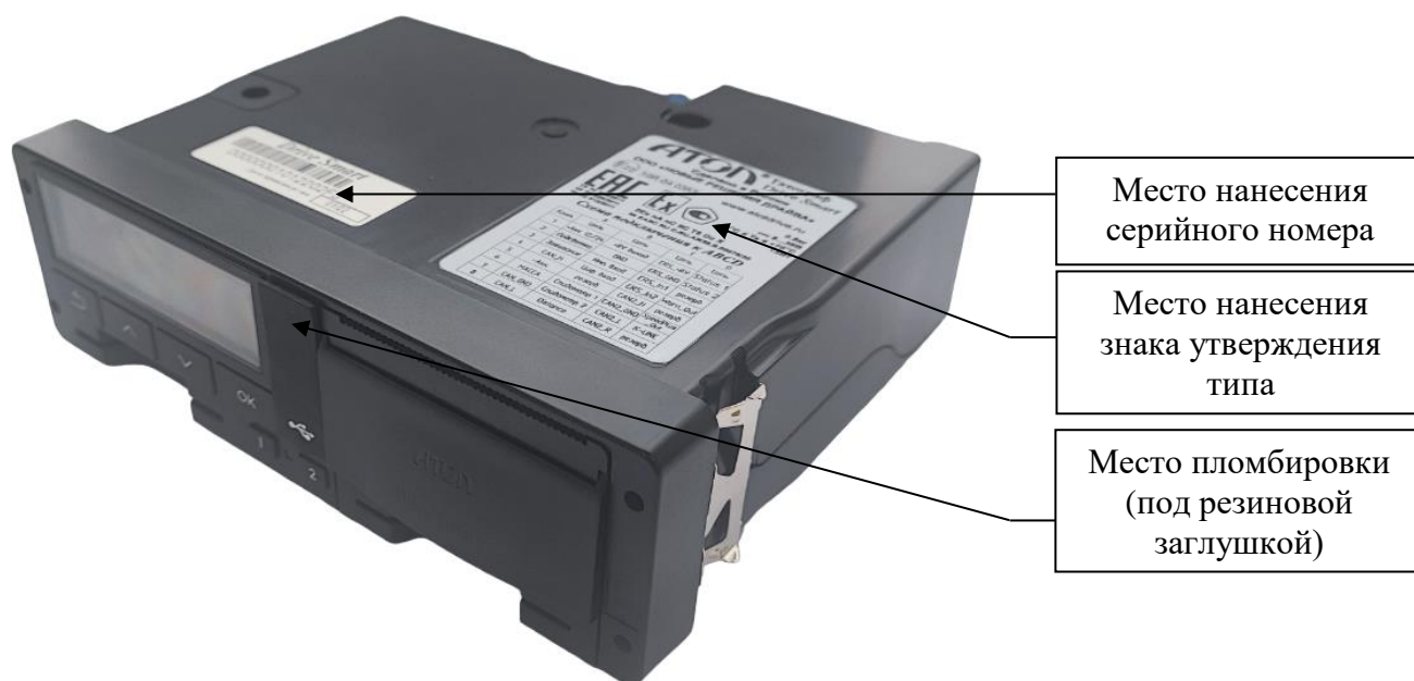
Рисунок 1 – Общий вид тахографов модификации Smart, выпускаемых под товарным знаком «АТОЛ»
