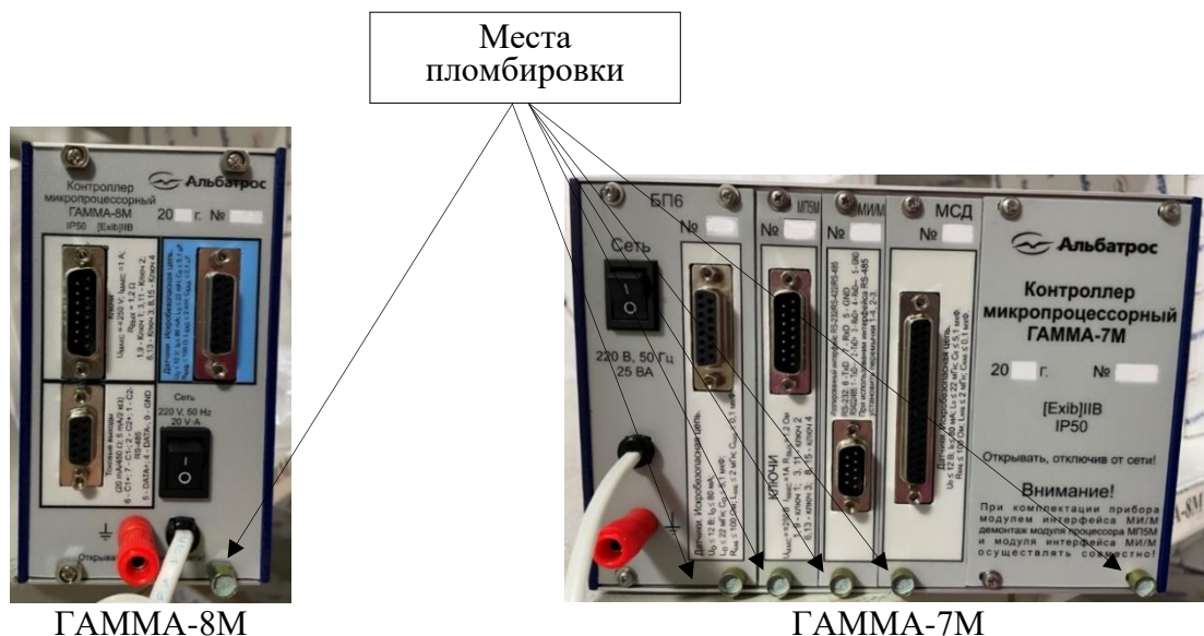
Рисунок 4 – Места пломбировки
