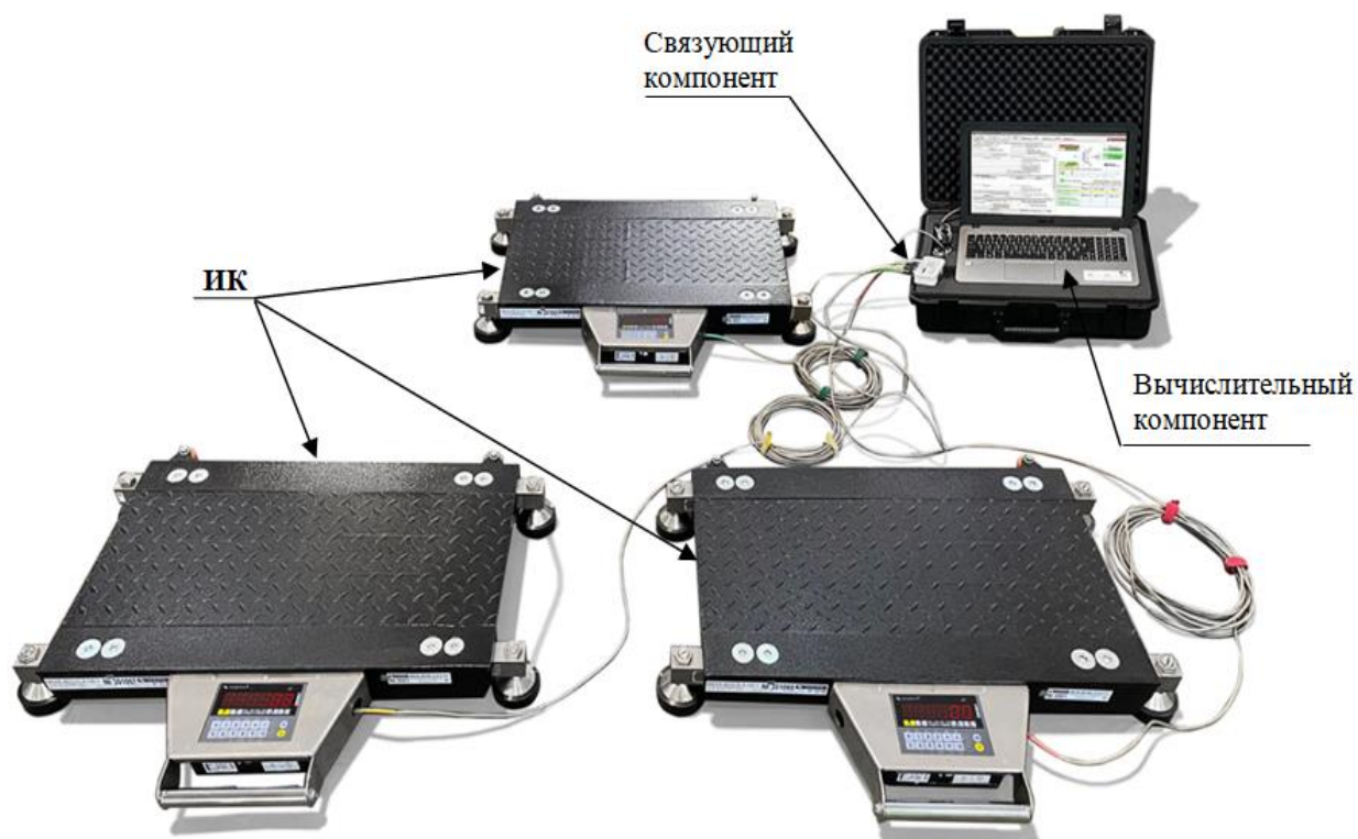
Рисунок 1 – Общий вид средства измерений (Z1=Π)
