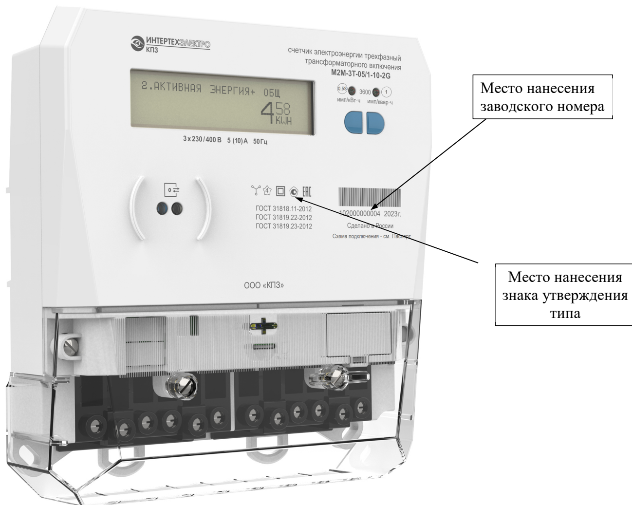
Рисунок 1 – Общий вид счетчика
