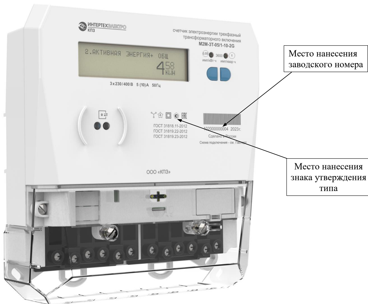
Рисунок 1 – Общий вид счетчика
