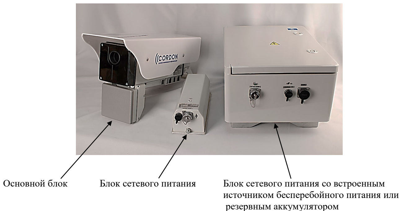
Рисунок 1 – Общий вид комплексов модификаций «Кордон.Про»МД-А и «Кордон.Про»МД-Р с блоками сетевого питания
