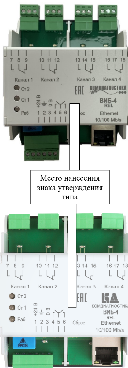
Рисунок 4 – Общий вид модуля исполнительных REL с указанием места нанесения знака утверждения типа
