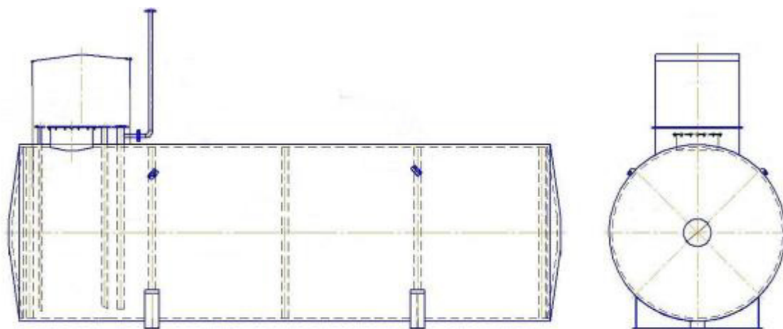
Рисунок 1 – Эскиз общего вида резервуаров РГС-25 зав.№№ 1, 4, 5, 8
