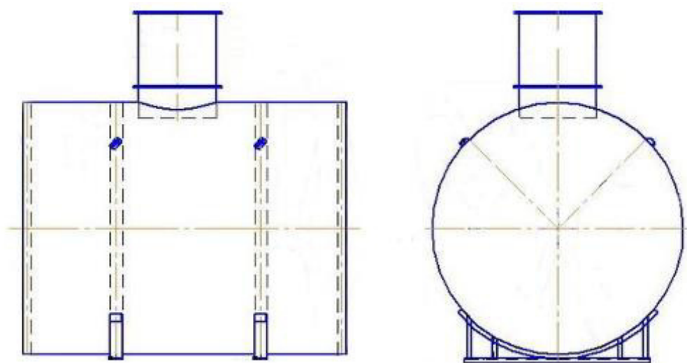
Рисунок 2 – Эскиз общего вида резервуаров РГС-25 зав.№№ 3, 6
