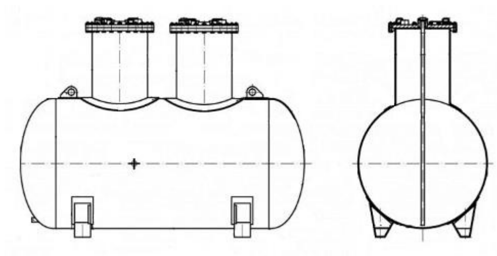
Рисунок 1 – Эскиз общего вида резервуаров РГС-50
