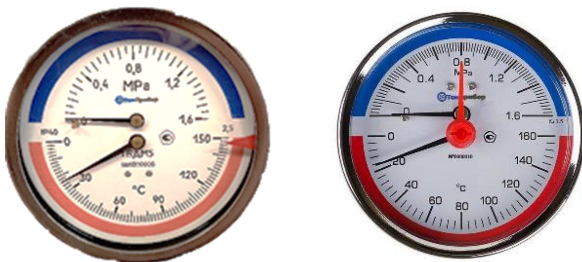
Рисунок 9 – Общий вид манометров показывающих деформационных МТ с функцией измерения температуры (термоманометров) модификации ТБДМ
