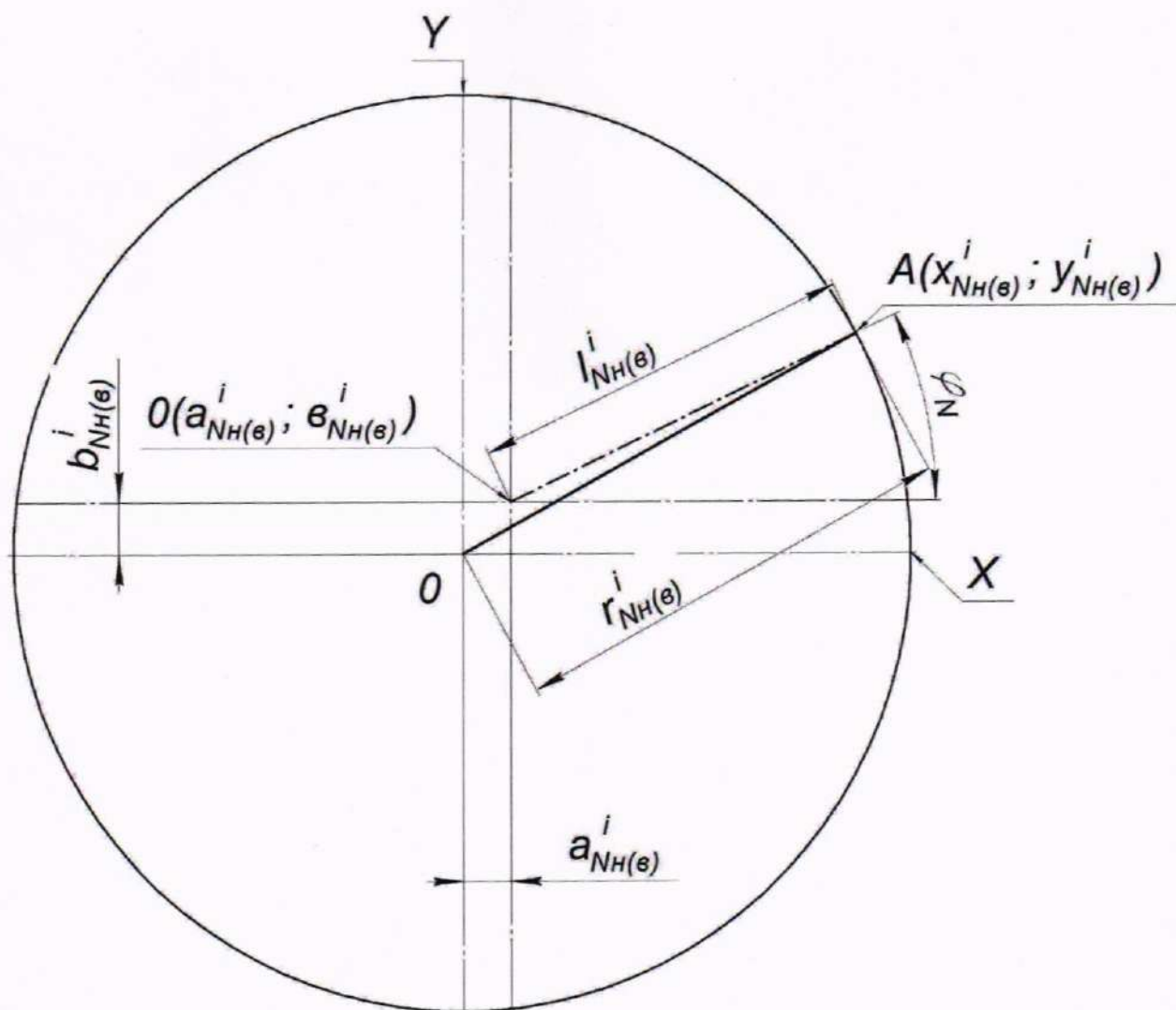
Рисунок Г.1 – Параметры измерений радиуса r_{NH(с)}^i i -го пояса при j -ом измерении в нижнем (верхнем) сечении
