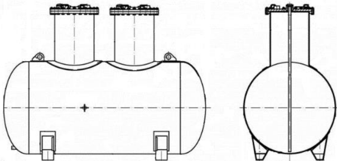
Рисунок 1 – Эскиз общего вида резервуаров РГС-60
