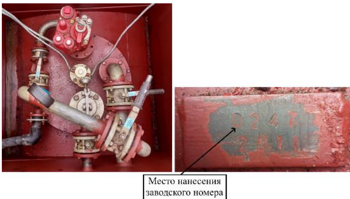
Рисунок 9 – Горловина и измерительный люк резервуара РГСД-25 зав.№ 0247
