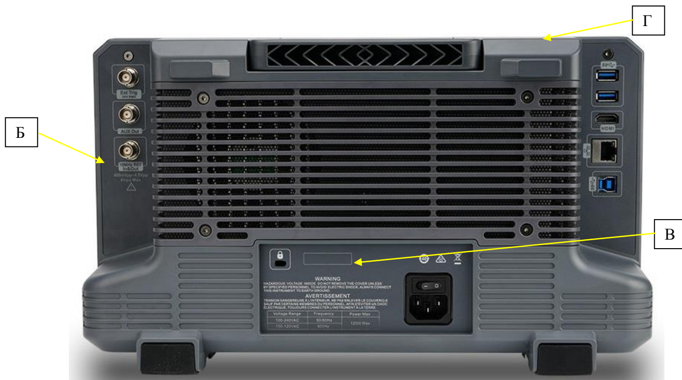
Рисунок 2 – Вид задней панели осциллографов, место пломбировки от несанкционированного доступа (Б), место нанесения серийного номера (В) и знака поверки (Г)
