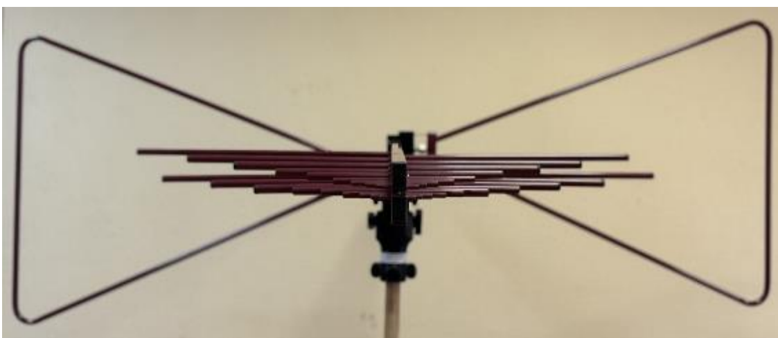
Рисунок 3 – Общий вид антенны BME-LB 9163
