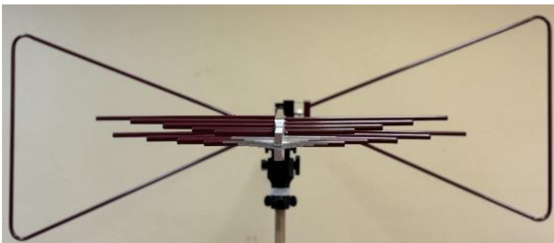
Рисунок 2 – Общий вид антенны BME-LB 9162
