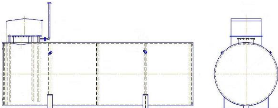
Рисунок 1 – Эскиз общего вида резервуаров РГС-25 зав. №№ 1, 2, 3, 5, 6
