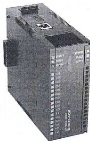
в) Модификация S-300-AO8
