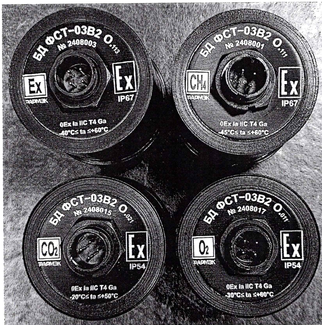
Рисунок 1.1 – Фотографии общего вида и маркировки БД ФСТ-03В2 О (изображение носит иллюстративный характер)
