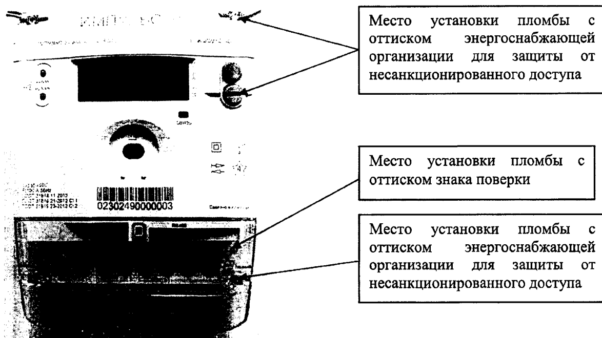
Рисунок 1 –Общий вид счетчика и схема пломбировки от несанкционированного доступа в корпусе типа W31
