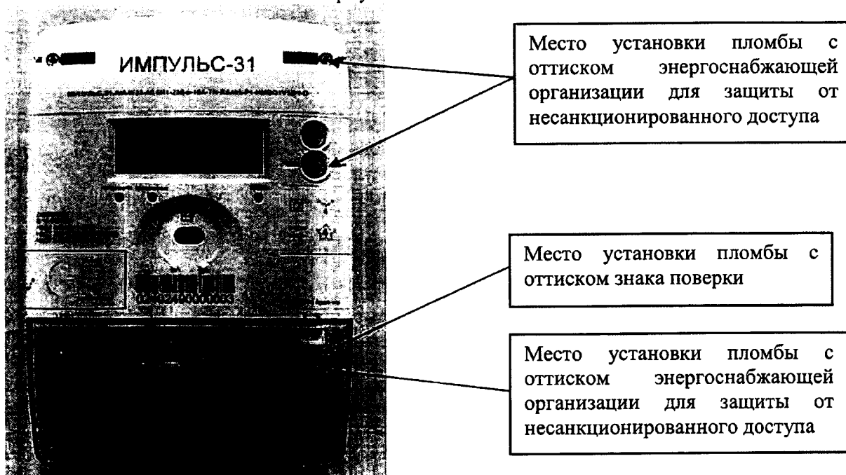
Рисунок 3 – Общий вид счетчика и схема пломбировки от несанкционированного доступа в корпусе типа W33
