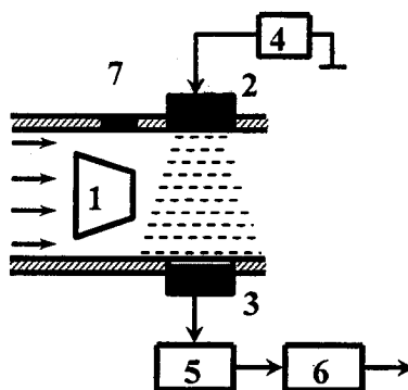
Рисунок 1.2 - Блок-схема преобразователя
