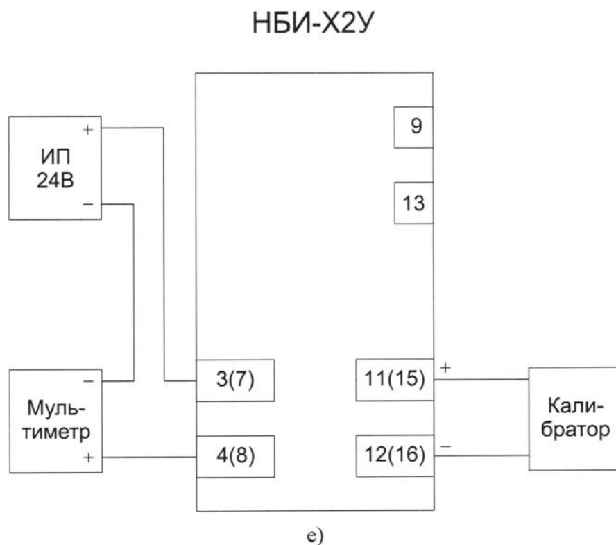
Рисунок А.1 Схемы подключения барьеров НБИ при опробовании и при определении основной приведенной к ДП погрешности преобразования силы постоянного тока в значения силы постоянного тока в рабочем диапазоне преобразования
