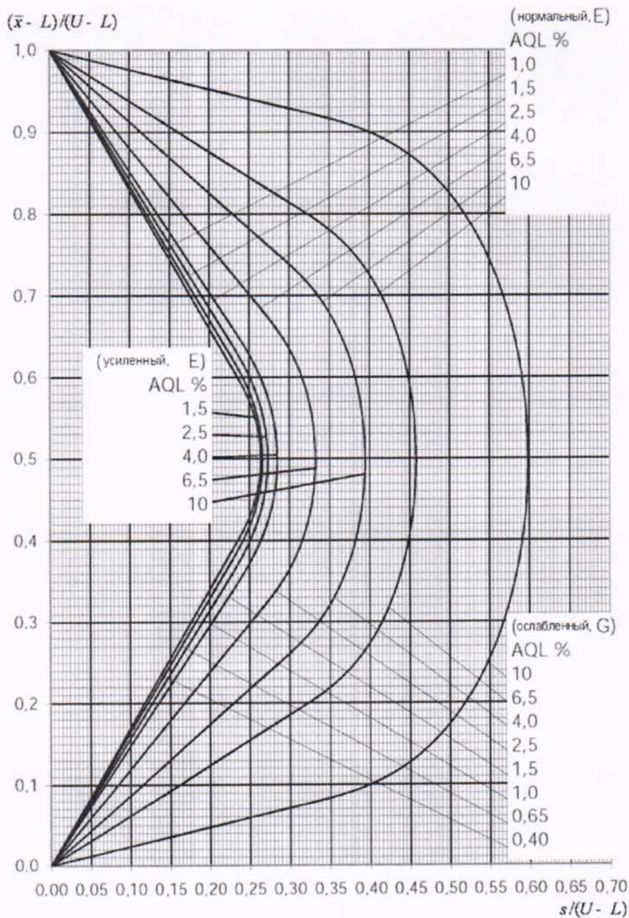
Рисунок Г.2 – График s-E. Приемочные кривые для объединенного контроля с двумя границами поля допуска для кода объема выборки E при нормальном и усиленном контроле и для кода
