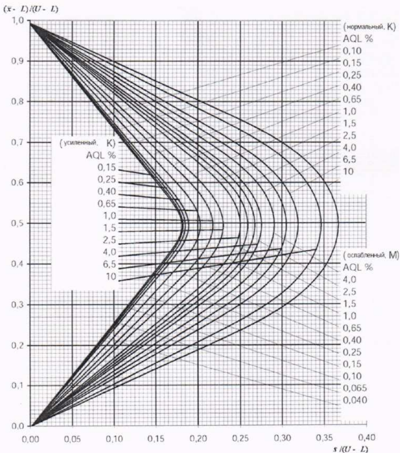
Рисунок Г.7 – График s-K. Приемочные кривые для объединенного контроля с двумя границами поля допуска для кода объема выборки K при нормальном и усиленном контроле и для кода объема выборки M при ослабленном контроле
