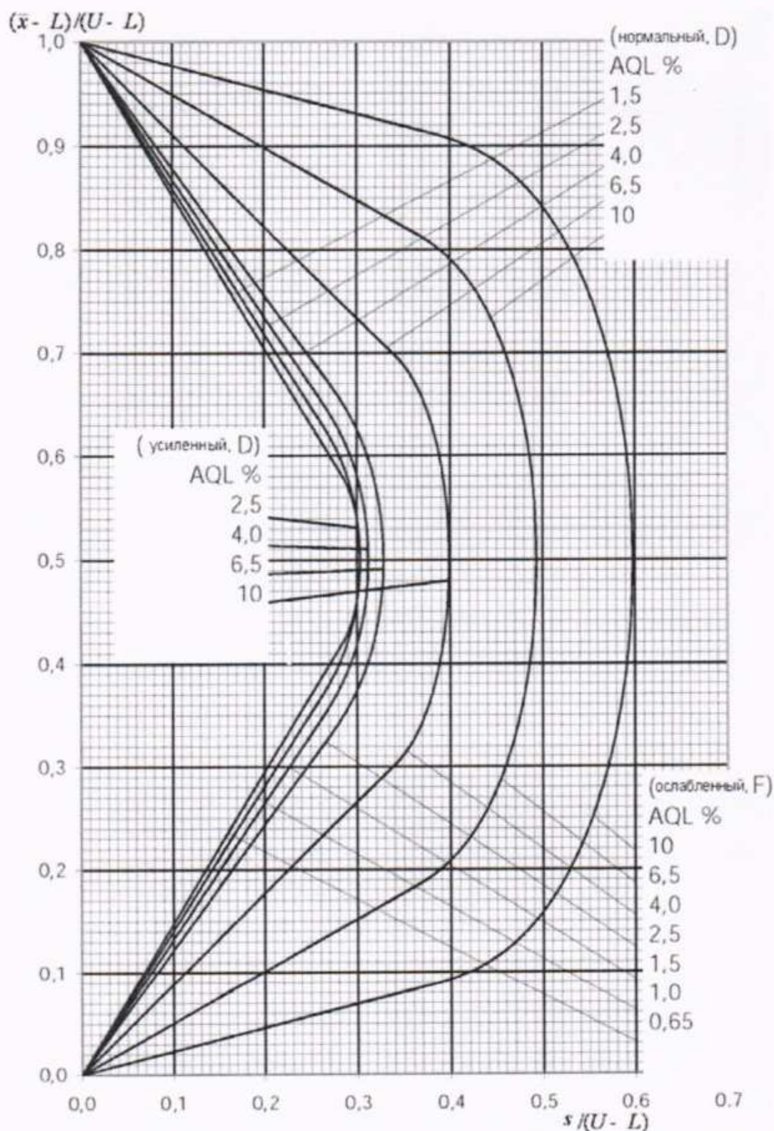
Рисунок Г.1 – График s-D. Приемочные кривые для объединенного контроля с двумя границами поля допуска для кода объема выборки D при нормальном и усиленном контроле и для кода объема выборки F при ослабленном контроле
