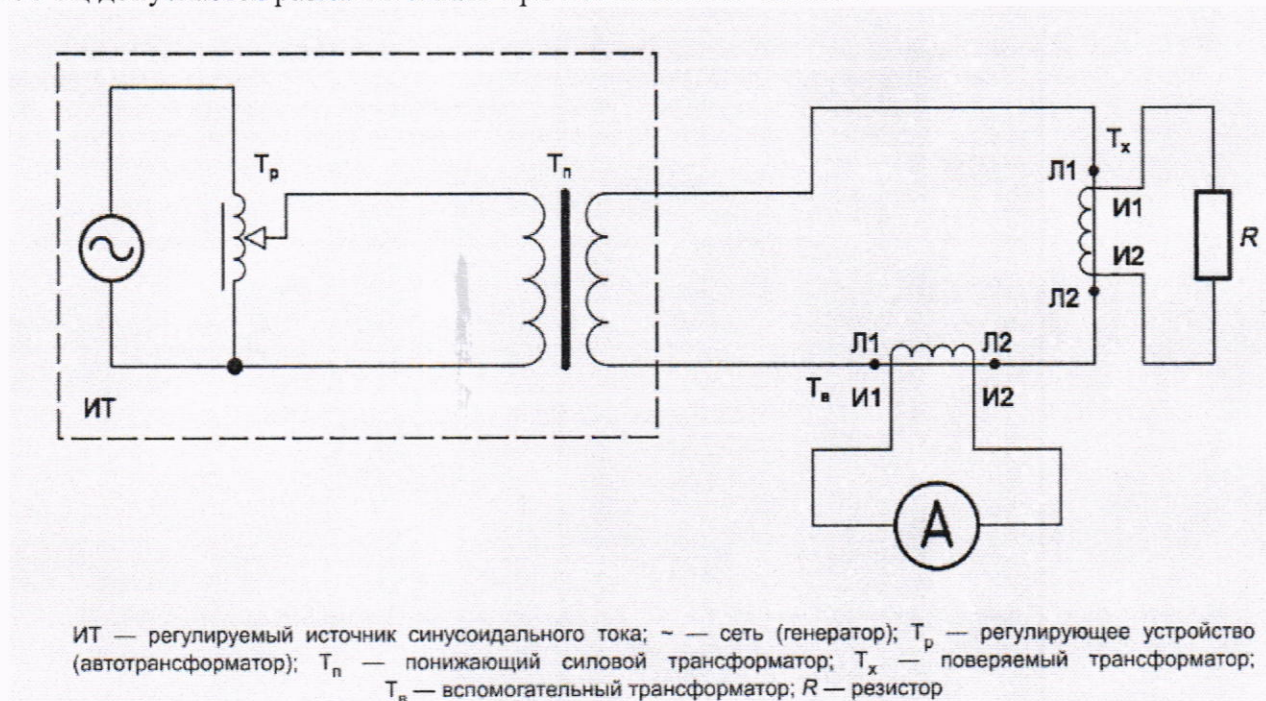
Рисунок 1 – Схема размагничивания трансформатора первым способом
