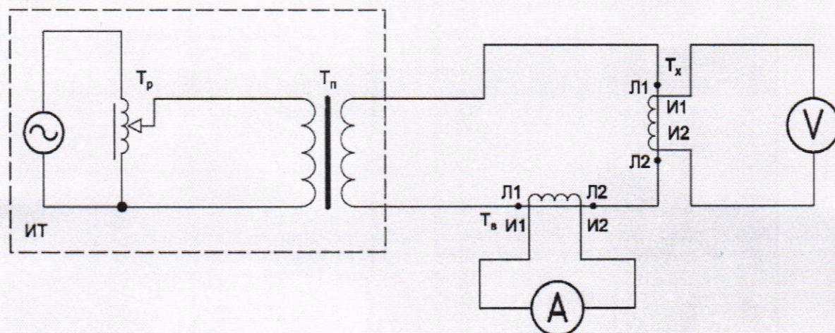
ИТ — регулируемый источник синусоидального тока; ~ — сеть (генератор); Т р — регулирующее устройство (автотрансформатор); Т п — понижающий силовой трансформатор; Т х — проверяемый трансформатор; Т в — вспомогательный трансформатор
