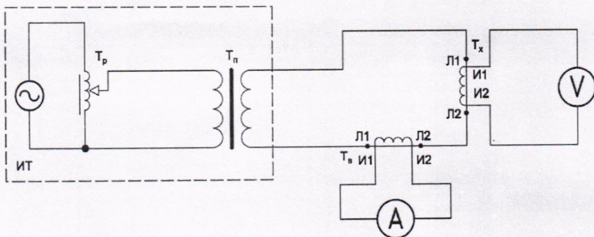
ИТ — регулируемый источник синусоидального тока; ~ — сеть (генератор); Т р — регулирующее устройство (автотрансформатор); Т н — понижающий силовой трансформатор; Т х — проверяемый трансформатор; Т в — вспомогательный трансформатор
