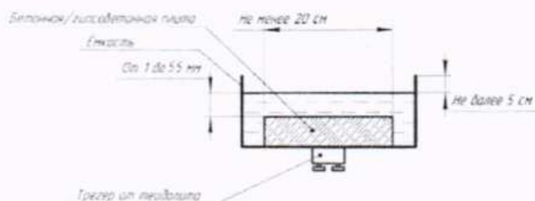
Рисунок Ж.1 – Емкость для измерений толщины слоя снега ПИП HY-RSS11E
