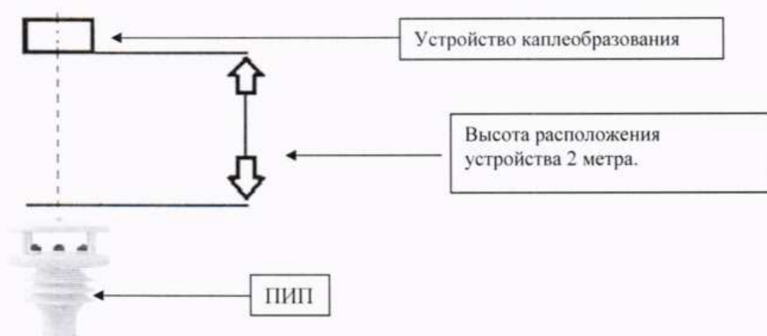
Рисунок 1 – Схема расположения устройства каплеобразования
