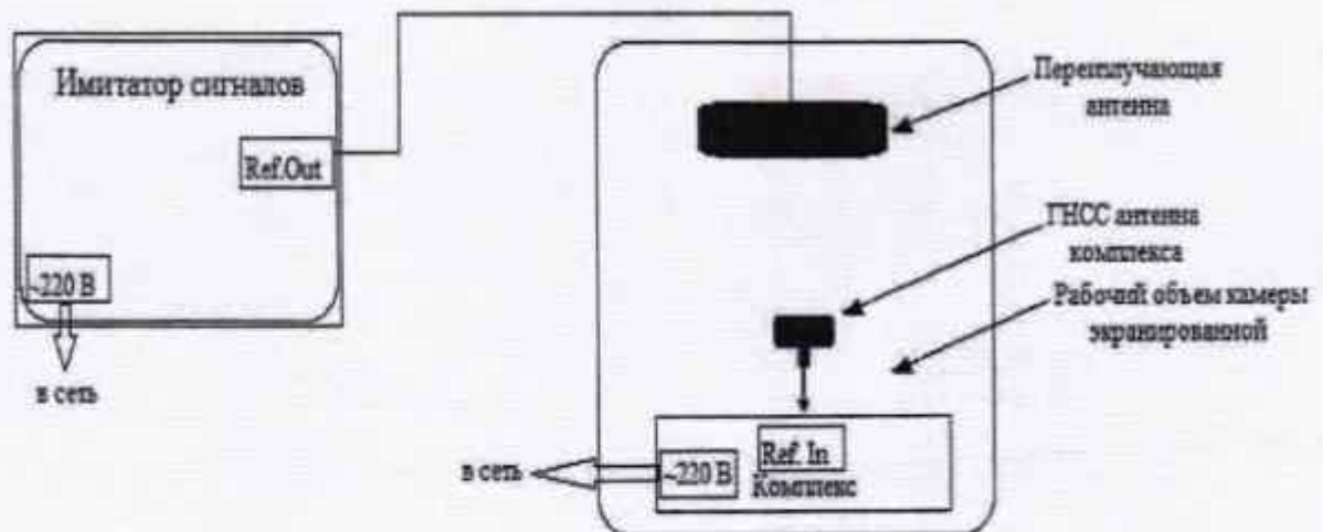
Рисунок 3 – Схема выполнения измерений
