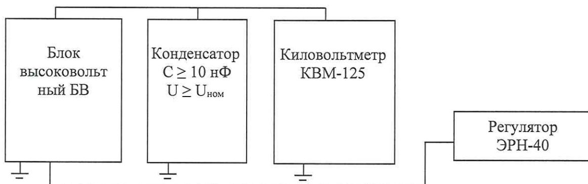
Рисунок 2 – Схема определения погрешностей на напряжении постоянного тока
