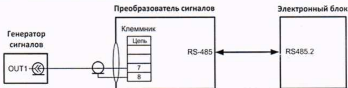
Рисунок 3 - Схема подключения к блоку ПС
