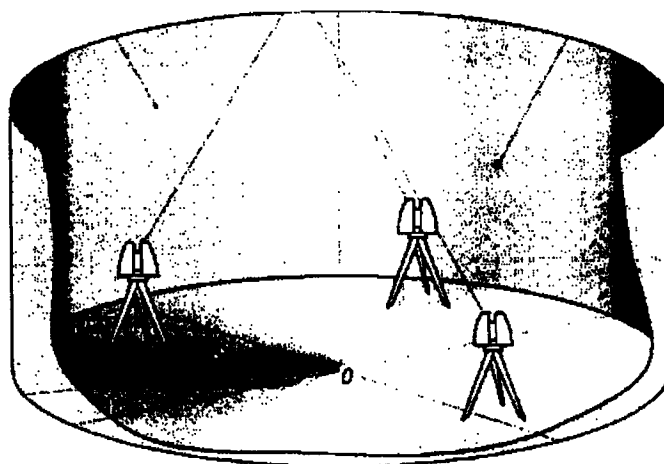
Рисунок А.2 - Схема сканирования внутренней полости резервуара
