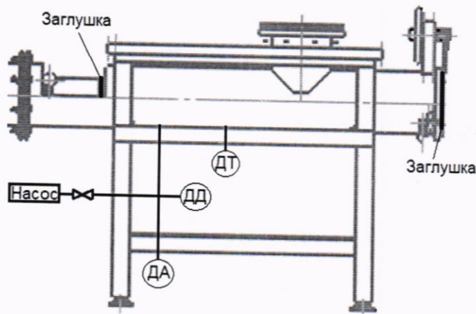
Рисунок 1 – Схема проверки герметичности.
