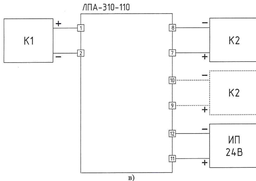
Рисунок А.1 Схемы подключения повторителей ЛПА-310 при опробовании и определении основной приведенной к ДП погрешности преобразования силы постоянного тока в значения силы постоянного тока в рабочем диапазоне преобразования
