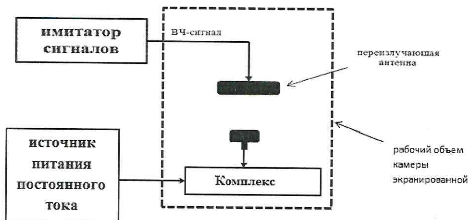
Рисунок 7 – Схема выполнения измерений
