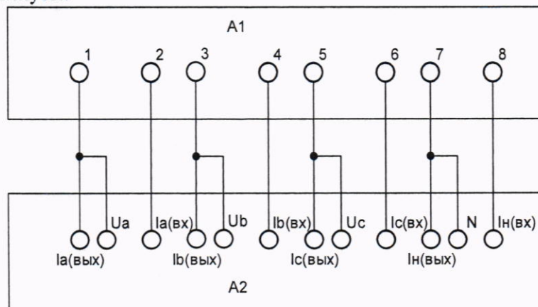
Рисунок 1 – Схема подключения счетчика к поверочной установке
