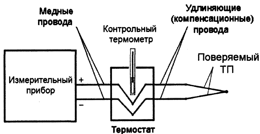
Рисунок 3 – Схема подключения, поверяемого ТП к измерительному прибору
