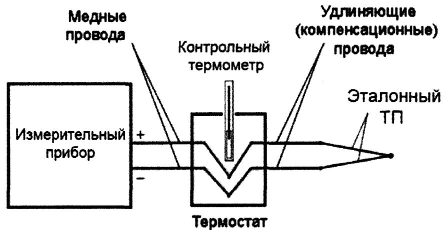
Рисунок 2 - Схема подключения эталонного ТП к измерительному прибору
