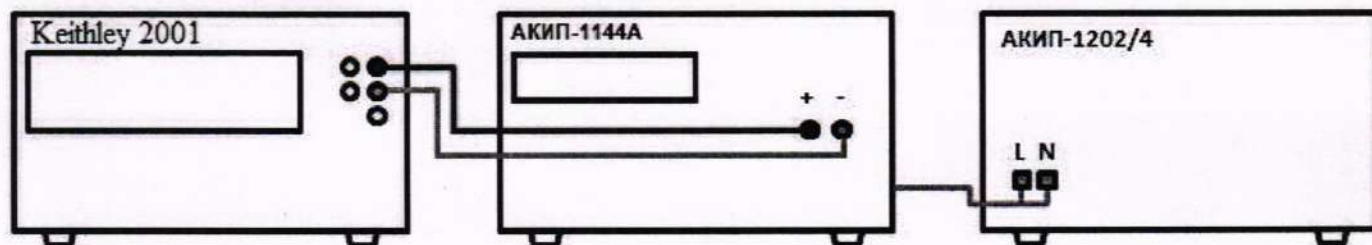
Рисунок 1 – Схема соединения приборов при определении пределов допускаемой основной абсолютной погрешности воспроизведения напряжения постоянного тока
