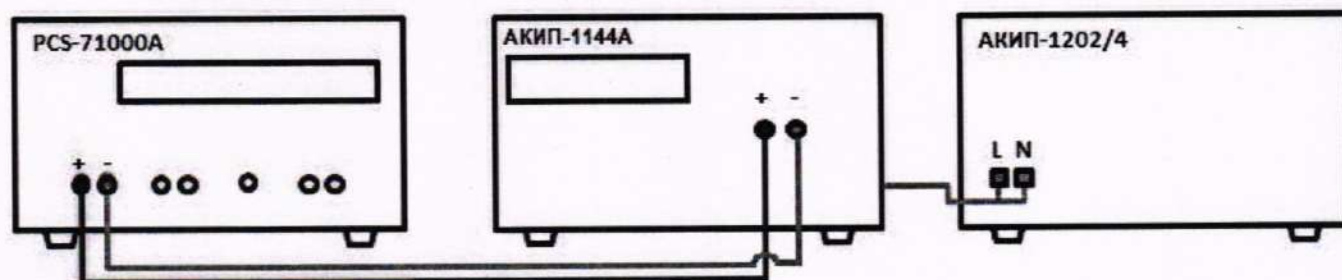
Рисунок 2 – Схема соединения приборов при определении пределов допускаемой основной абсолютной погрешности воспроизведения силы постоянного тока
