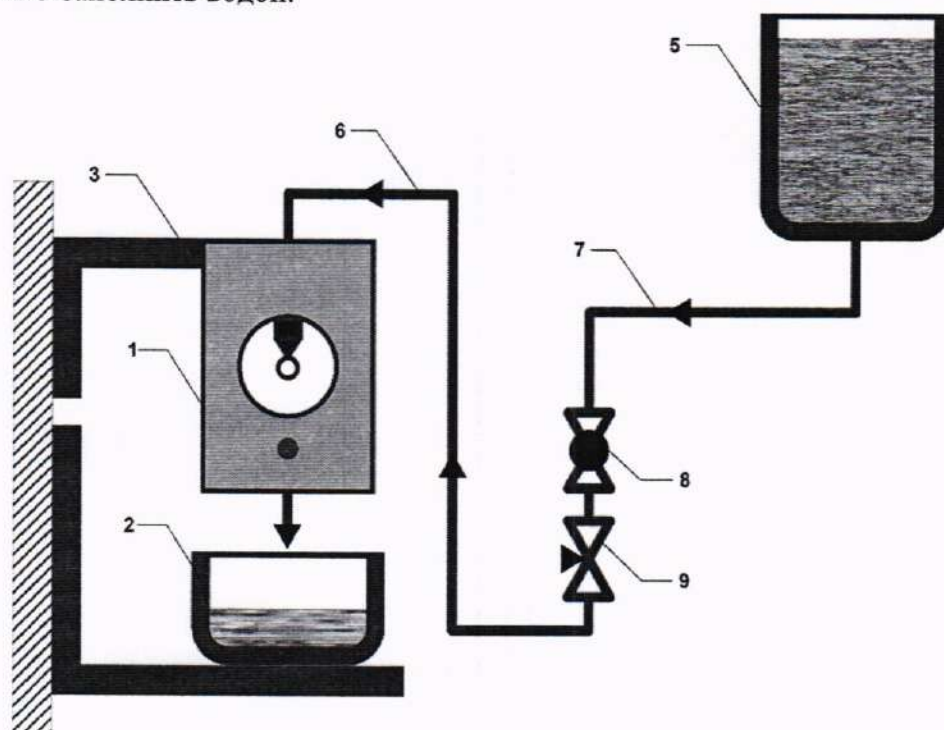
Рис. 1 - Подготовка датчика расхода воды.
