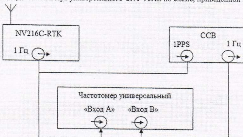
Рисунок 2 – Схема определения допускаемой абсолютной погрешности привязки переднего фронта выходного импульса частотой 1 Гц к сигналам внешней синхронизации 1PPS
