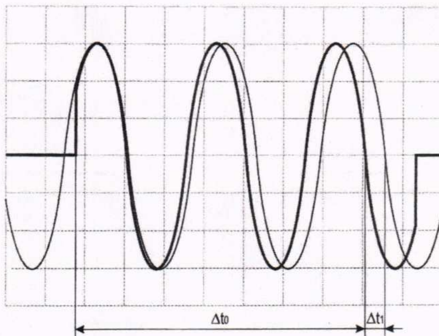
Рисунок 1 – Осциллограмма работы реле «Синхро» при опережении срабатывания реле К1 равным 0
