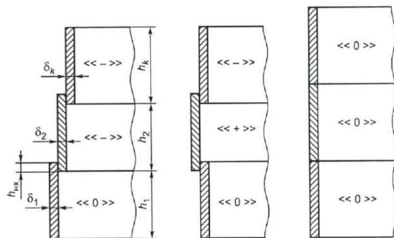
а) Телескопическая б) Комбинированная в) Встык
