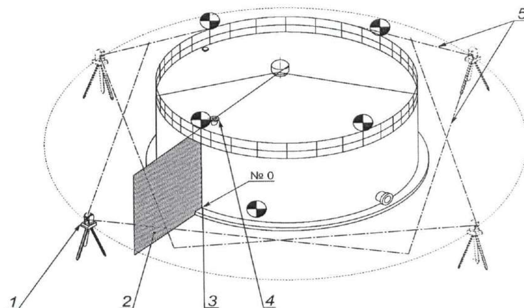
Рисунок А.5 – Схема сканирования внутренней полости резервуара с плавающим покрытием
