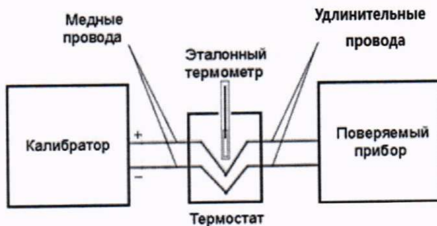
Рисунок 1 – Схема подключения
