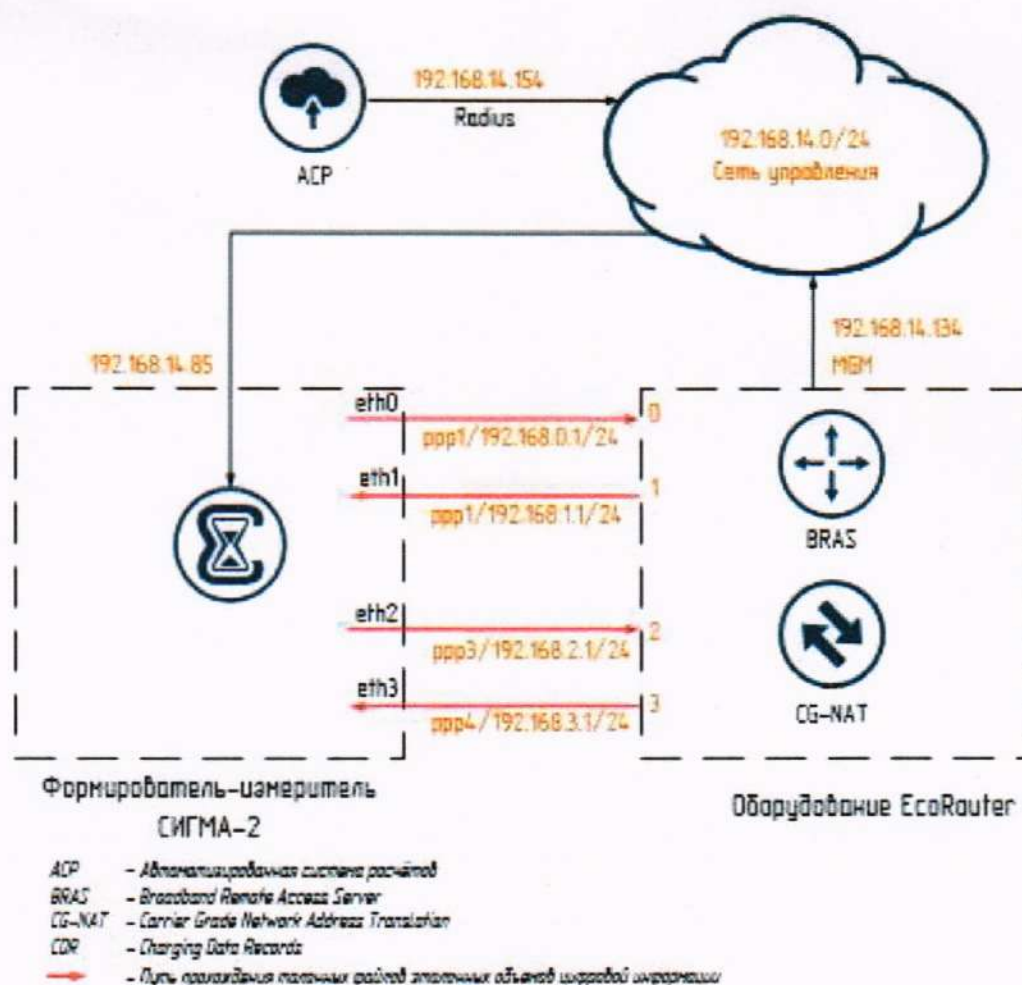
Рисунок 1 – Схема поверки СИПД
