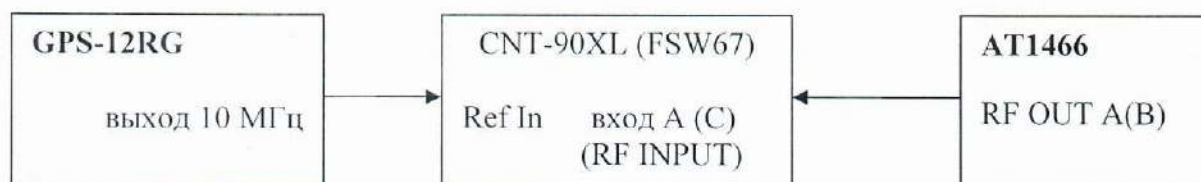
Рисунок 1 – Структурная схема соединения СИ для определения относительной погрешности установки частоты при работе от внутреннего опорного генератора
