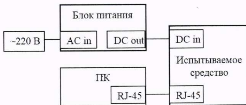
Рисунок 3 – Схема проведения измерений
