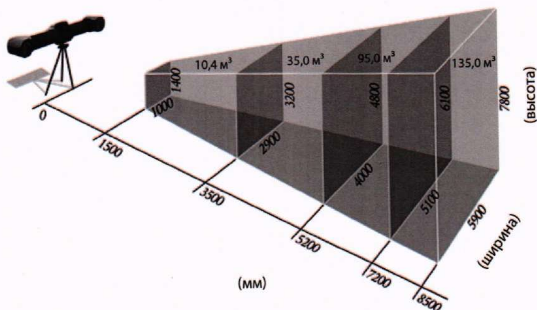
Рисунок А.1 – Схема измерительного объема системы
