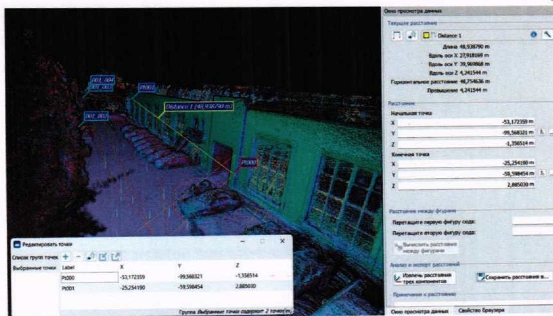
Рисунок 3 – Отображение значений приращений координат в программном обеспечении
