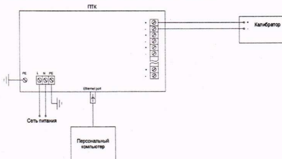
Рисунок 5 – Схема подключений при определении приведенной к диапазону воспроизведений погрешности воспроизведений силы постоянного тока
